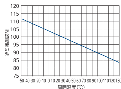
図5. ブレードヒューズの温度変化率
