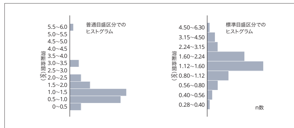
図7. 溶断時間のバラツキ
