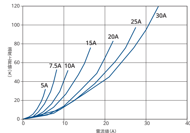
図2. 温度上昇
