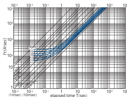
図6. I^2t 特性図
