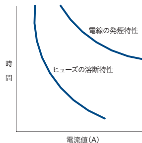
図8. ヒューズの溶断特性と電線の発煙特性
