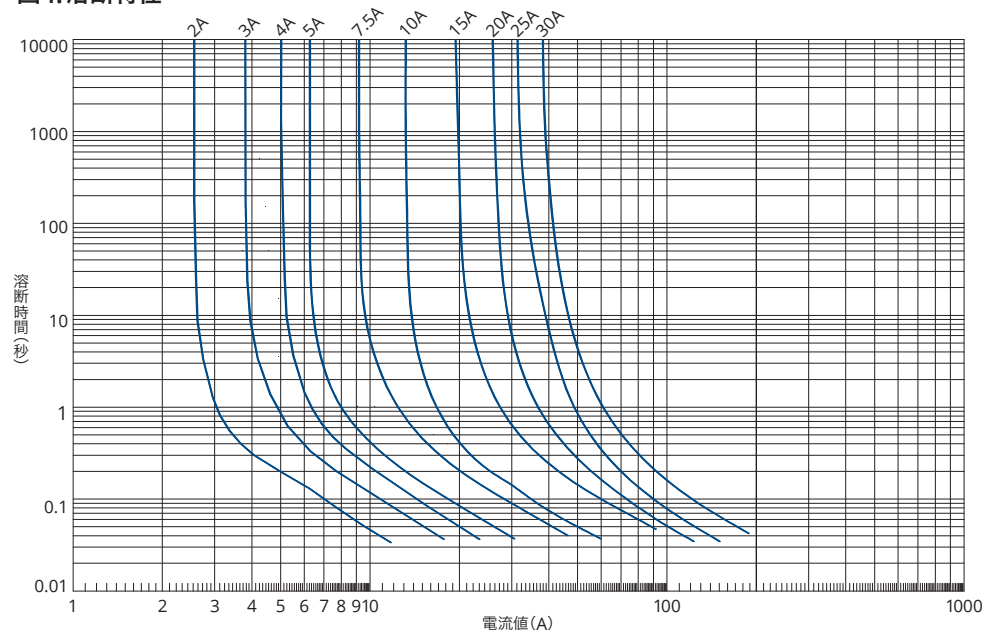
図4. 溶断特性
